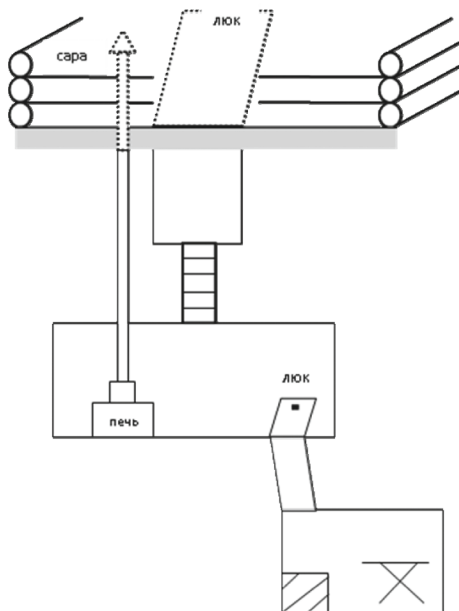
Схема расположения и устройство бункера в районе хутора Хала (Бункер обнаружен ротой под командованием старшего лейтенанта Добренького).
