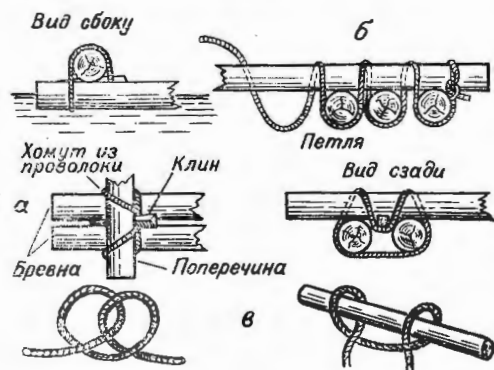
Рис. 2. Вязание плота из длинных бревен: а — крепление бревен к поперечинам проволокой; б — крепление бревен канатами «впереплет»; в — найтовый узел.
