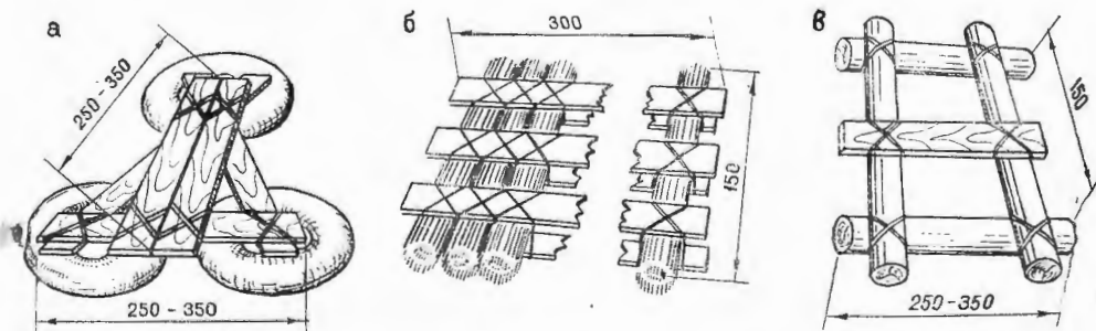
Рис. 1. Переправы на 1—2 человек:
