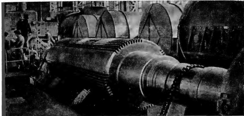
Обработка тяжеловесного (150 тонн, диаметр 1,8 метра) ротора четырехполюсного «миллионника» на специальном роторно-фрезерном станке.
