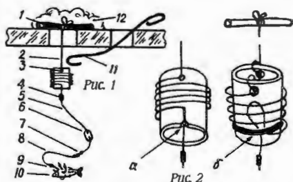
Рис. 1. Общий вид жерлицы в рабочем положении.
